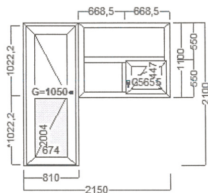
Poz: 4 [stijena sa dvokrilnim prozorom ( WC)] Km 1
