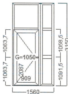
Poz : 18 [stijena sa prozrom ( SOBA 16)]
